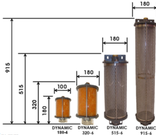
Acotación: mm
